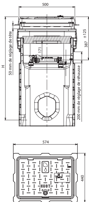
Poids Tête (cadre et tampon) : 17,5 Kg
