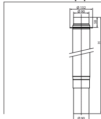
86/8 - Allonge tabernacle télescopique
