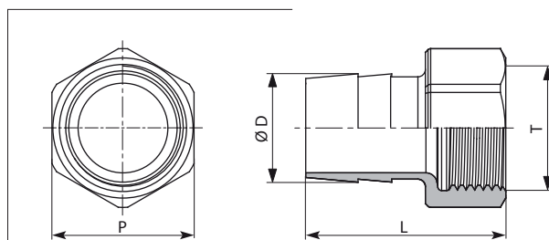
SR412/F - Raccord cannelé femelle
