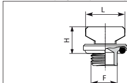
9/S - Bouchon purgeur à joint torique
