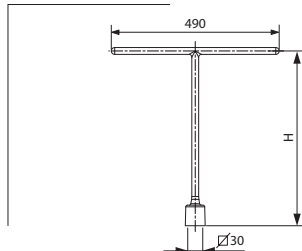
86/3 - Allonge PVC pour bouche à clé
