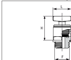
9/E - Robinet à orifice avec vis porte clapet imperdable
