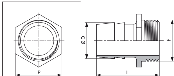
SR412 - Raccord cannelé mâle
