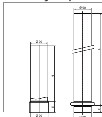
86/3-8 - Tube télescopique
