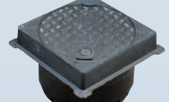
B : Tampon fonte B125 EN124 à verrou
